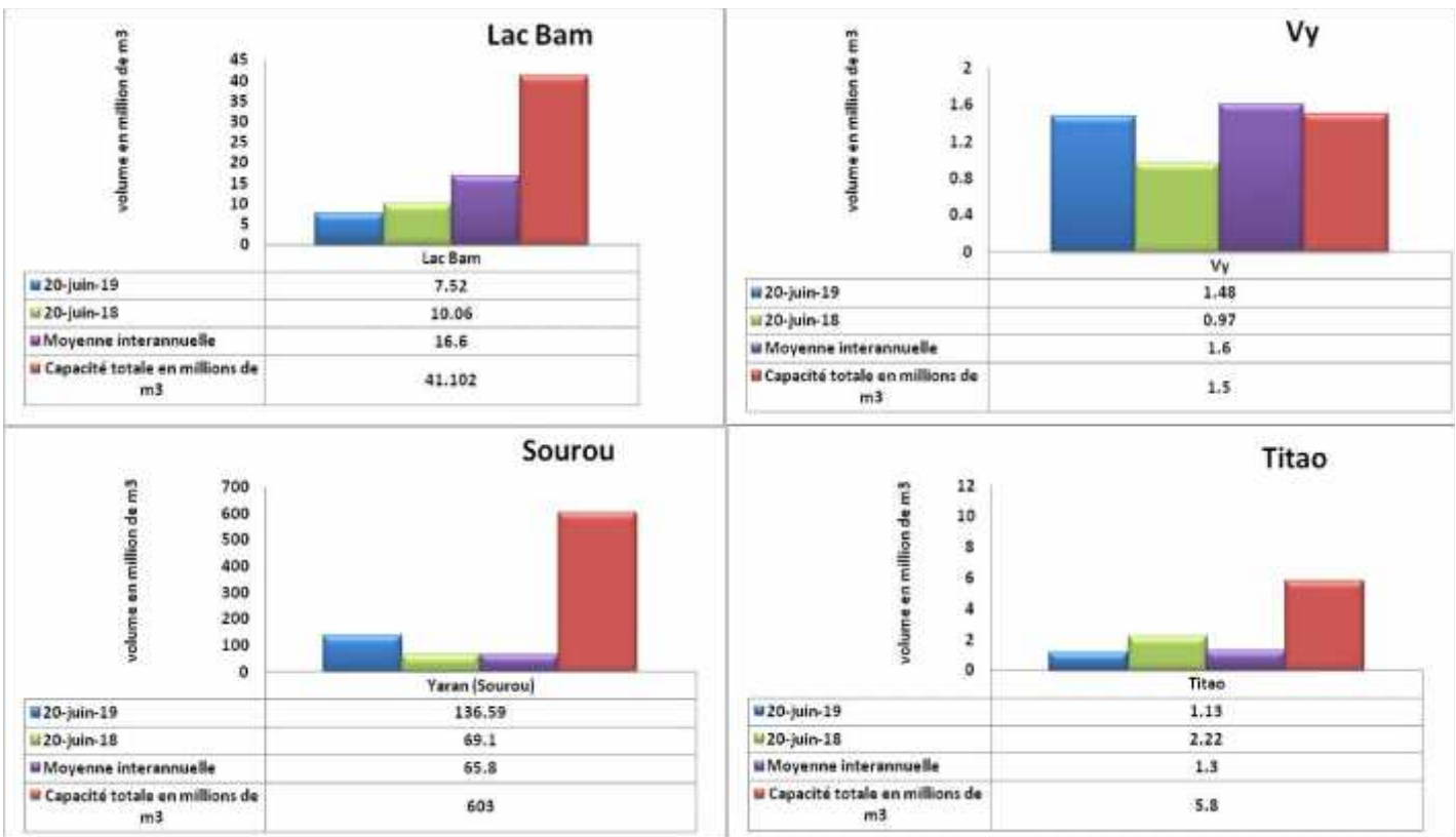
Figure 6 : Situation de remplissage au 20 juin 2019, comparaison avec la situation de 2018, la moyenne inter-annuelle et la capacité nominale des barrages.
