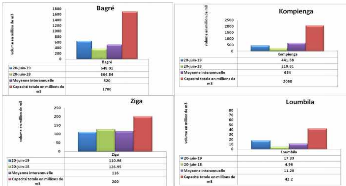
Figure 4 : Situation de remplissage au 20 juin 2019, comparaison avec la situation de 2018, la moyenne interannuelle et la capacité nominale des barrages.
