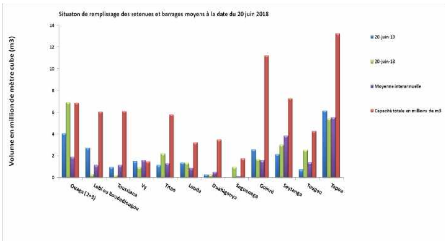
Figure 3 : Situation de remplissage au 20 juin 2019, comparaison avec la situation de 2018, la moyenne interannuelle et la capacité nominale des barrages.
