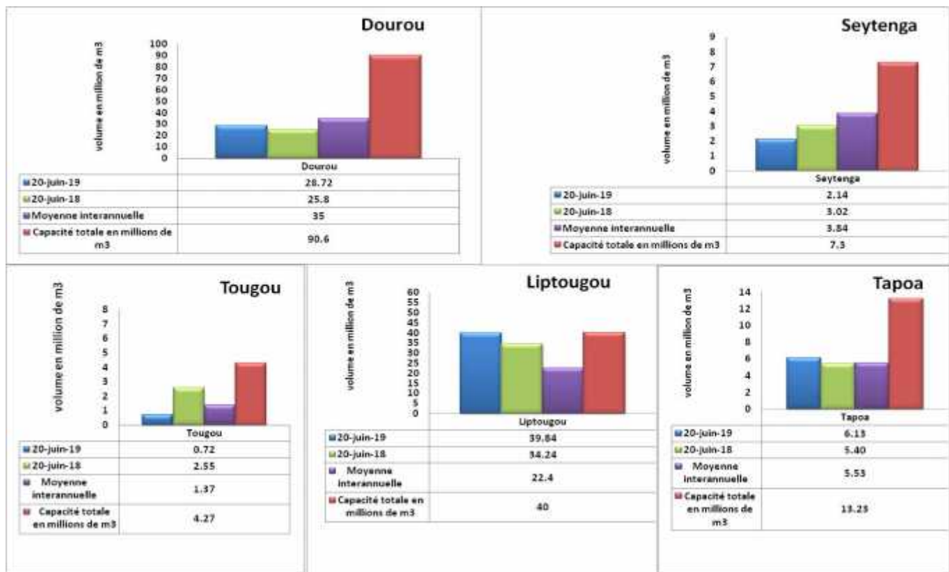
Figure 8 : Situation de remplissage au 20 juin 2019, comparaison avec la situation de 2018, la moyenne interannuelle et la capacité nominale des barrages.
