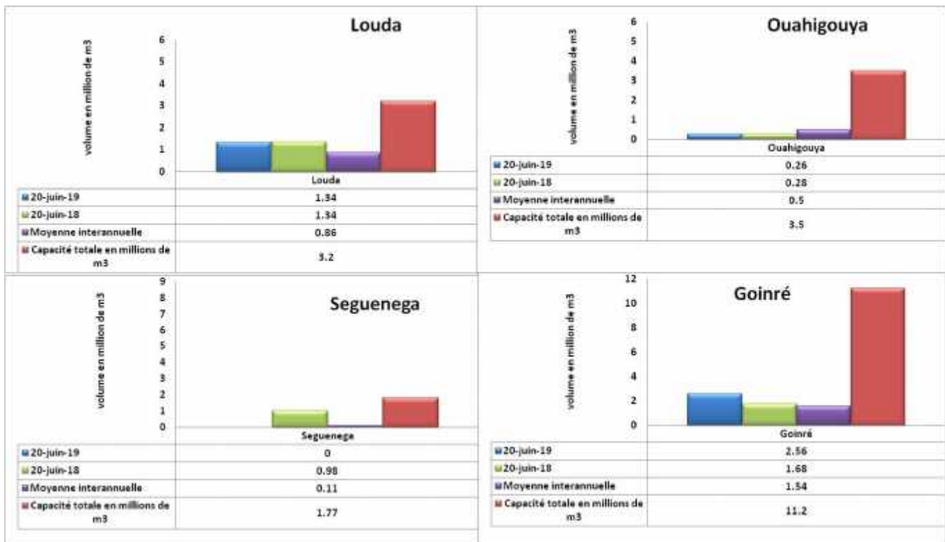
Figure 7 : Situation de remplissage au 20 juin 2019, comparaison avec la situation de 2018, la moyenne interannuelle et la capacité nominale des barrages.
