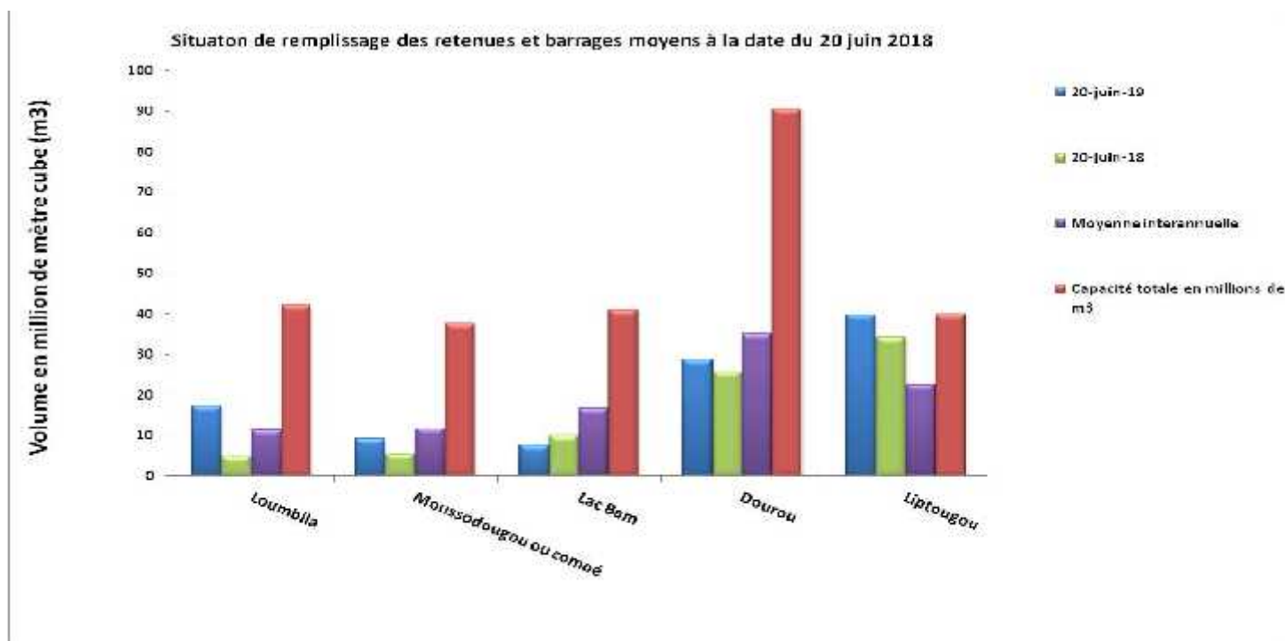
Figure 2: Situation de remplissage au 20 juin 2019, comparaison avec la situation de 2018, la moyenne inter-annuelle et la capacité nominale des barrages.
